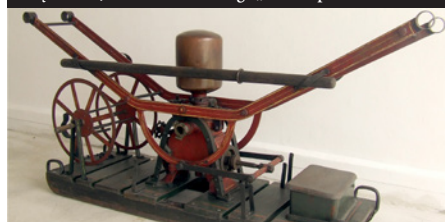
Sikawka przenośna 1-cylindrowa „Tryumf” z 1927 r. Dar OSP Lipiny, gm. Mrozy, dla MPK w dniu 9.10.1983 r.
